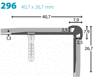
Trapneus met inschuif Aluminium. Voor vloerhoogte 2,5 mm. Verzonken geboord
