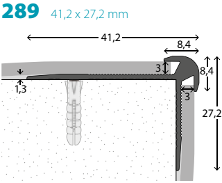
Trapneus met inschuif Aluminium. Voor vloerhoogte 3 mm. Verzonken geboord
