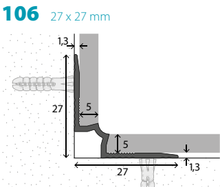
Binnenhoek Aluminium. Voor vloerhoogte 4-5 mm. Verzonken geboord
