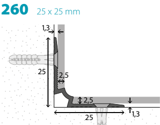
Binnenhoek Aluminium. Voor vloerhoogte 2-2,5 mm. Verzonken geboord
