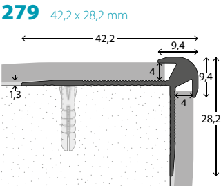
Trapneus met inschuif Aluminium. Voor vloerhoogte 3,2-4 mm. Verzonken geboord
