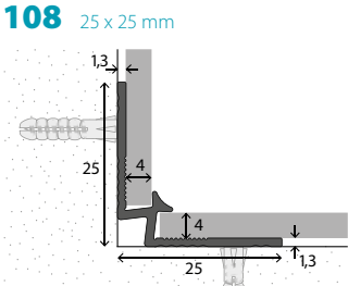
Binnenhoek met inschuif Aluminium. Voor vloerhoogte 3,2-4 mm. Verzonken geboord
