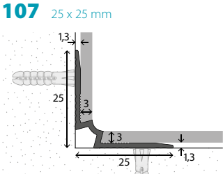
Binnenhoek Aluminium. Voor vloerhoogte 2,5-3 mm. Verzonken geboord
